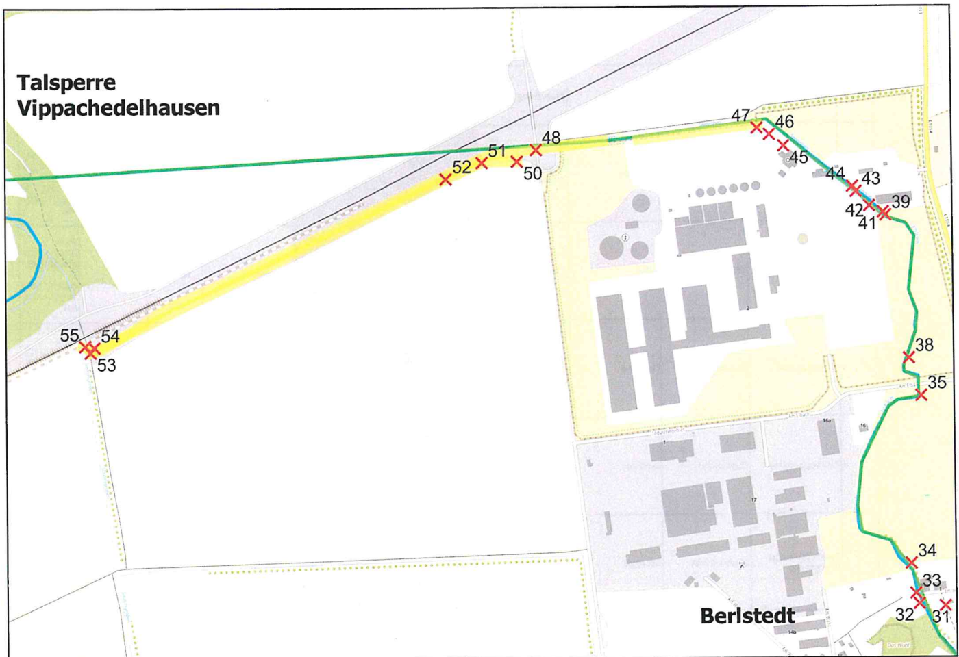
Abschnitt 3: von Ende Siedlungsbereich Berlstedt bis Einmündung in Sautalsgraben südlich Talsperre Vippachedelhausen
