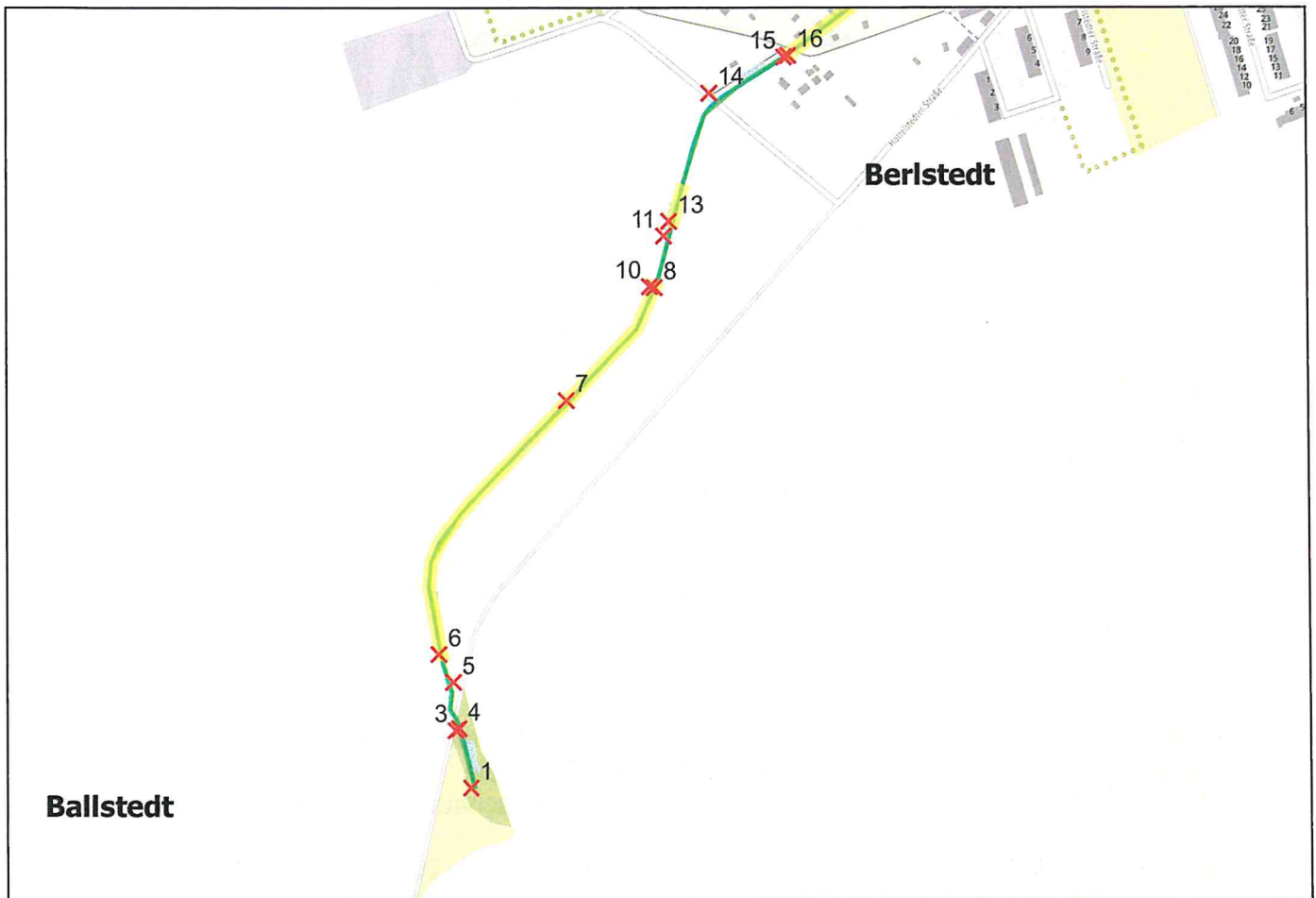
Abschnitt 1: von Beginn Ellgraben bis Beginn Verrohrung mit Einlaufrechen vor Kleingartenanlage im Süden Berlstedts
